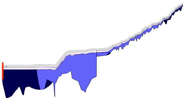
Figuur 2. Doorsnede van de hangende dam in St-Raymond. Stroomafwaarts de dam van de papierfabriek (rood), de ijslaag (wit) met daarbovenop sneeuw (grijs) en daaronder frazil (lichtblauw).
